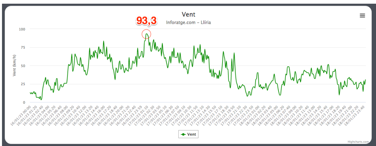
Ráfagas de viento registradas en LLÍRIA entre el 16 y el 18/01/23 https://inforatge.com/meteo-lliria
